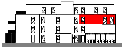
VOORGEVEL
